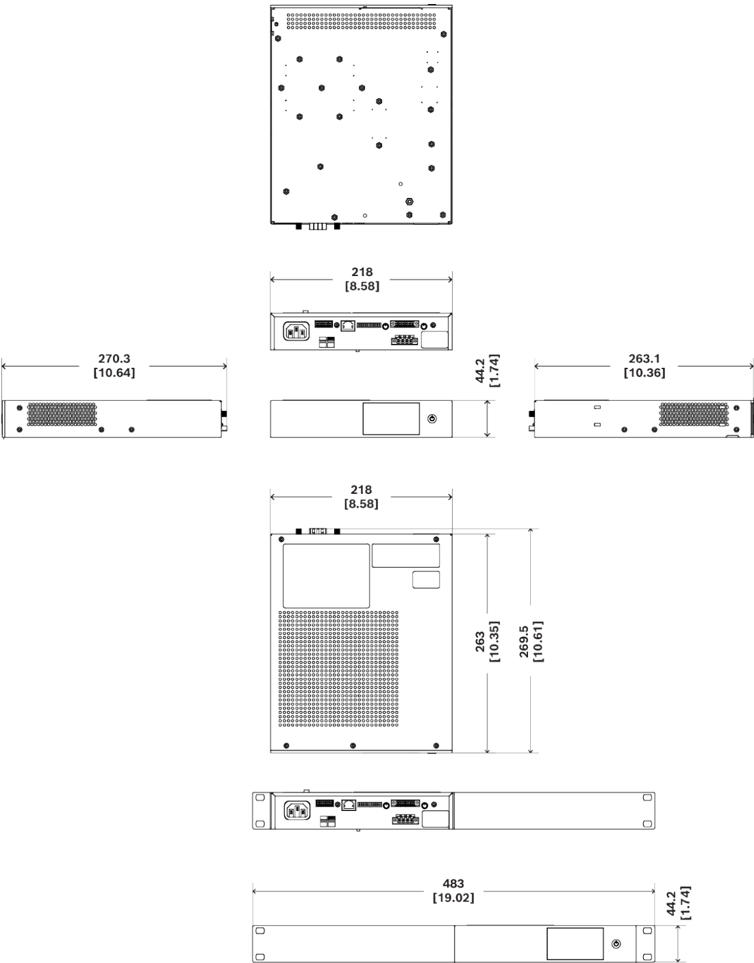
Fig. 3: Dimensions
