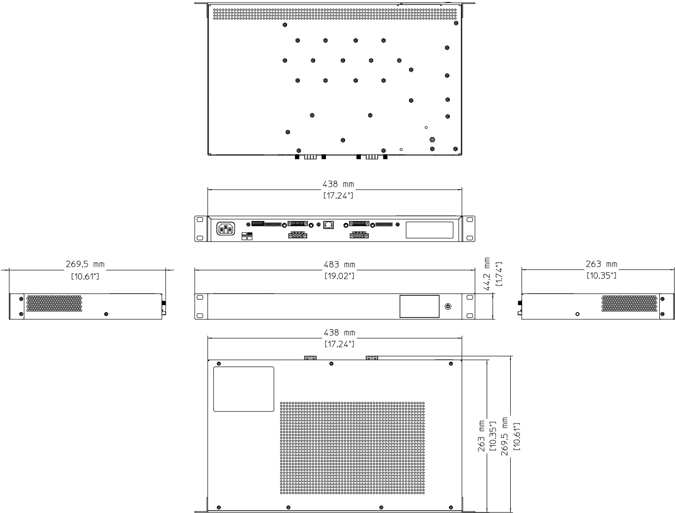
Fig. 3: Dimensions
