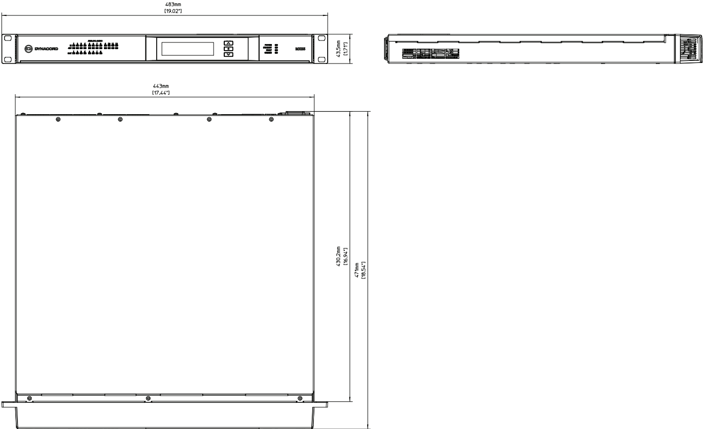
Fig. 2: Dimensions
