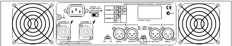
Q44, Q66, Q99 and Q1212 rear view
