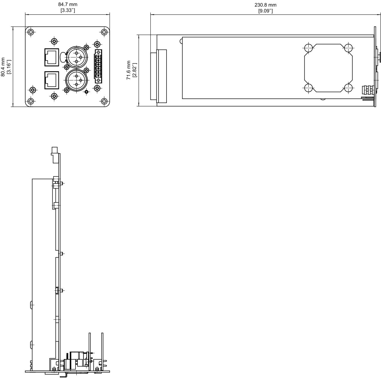
Dimensions
