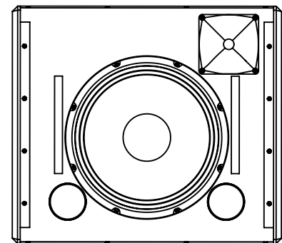
TOP - BAFFLE
