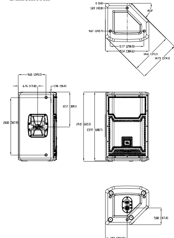
Dimensions
