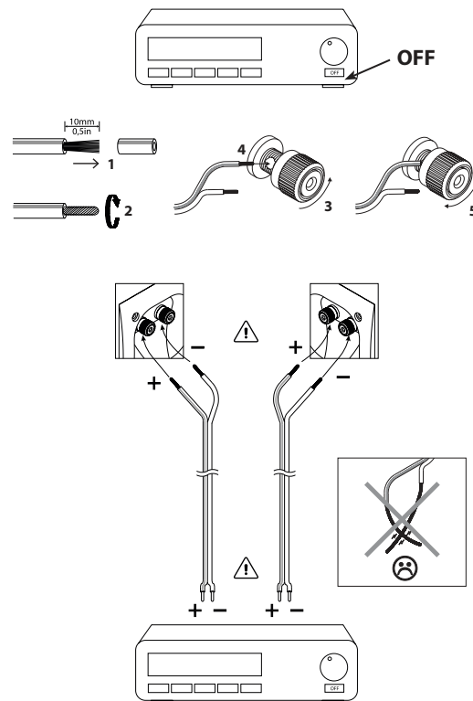
FIGURA 3 CONNESSIONI STANDARD
