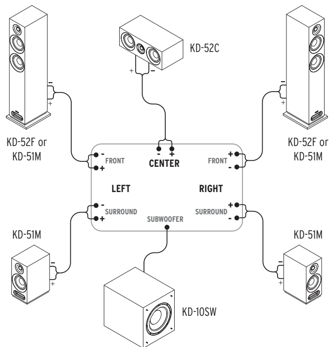
FIGURA 4 CONEXIONES ESTÁNDAR
