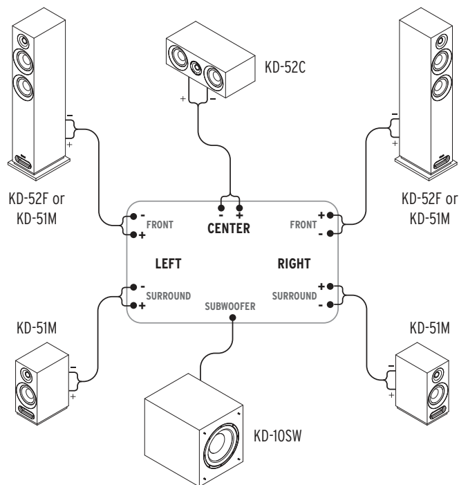
ABBILDUNG 4 STANDARDANSCHLÜSSE
