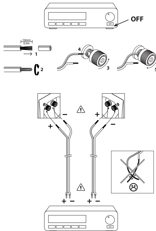
FIGURA 3 CONNECTIN CONEXIONES ESTÁNDAR
