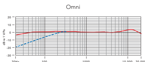
Omni
