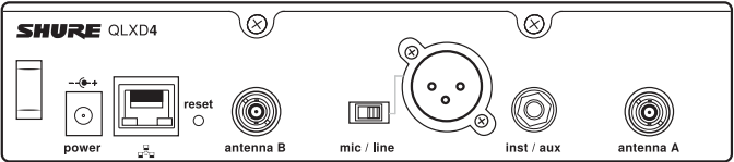
QLXD4 Back Panel
