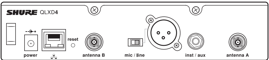
QLXD4 Back Panel
